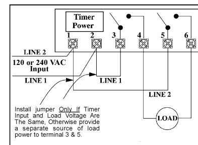
FIG. #4 ET173C DPST ET174C DPST
